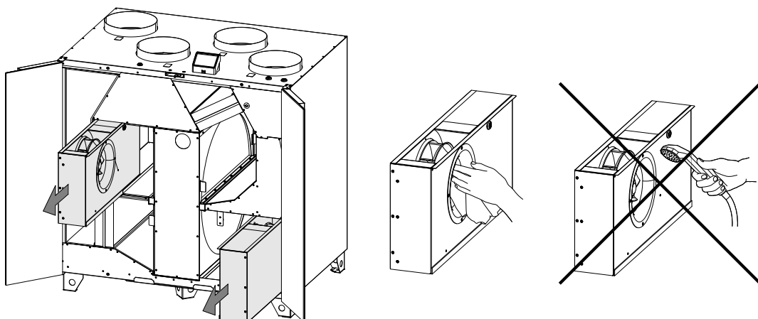
Fig. 6 De ventilatoren verwijderen en reinigen
