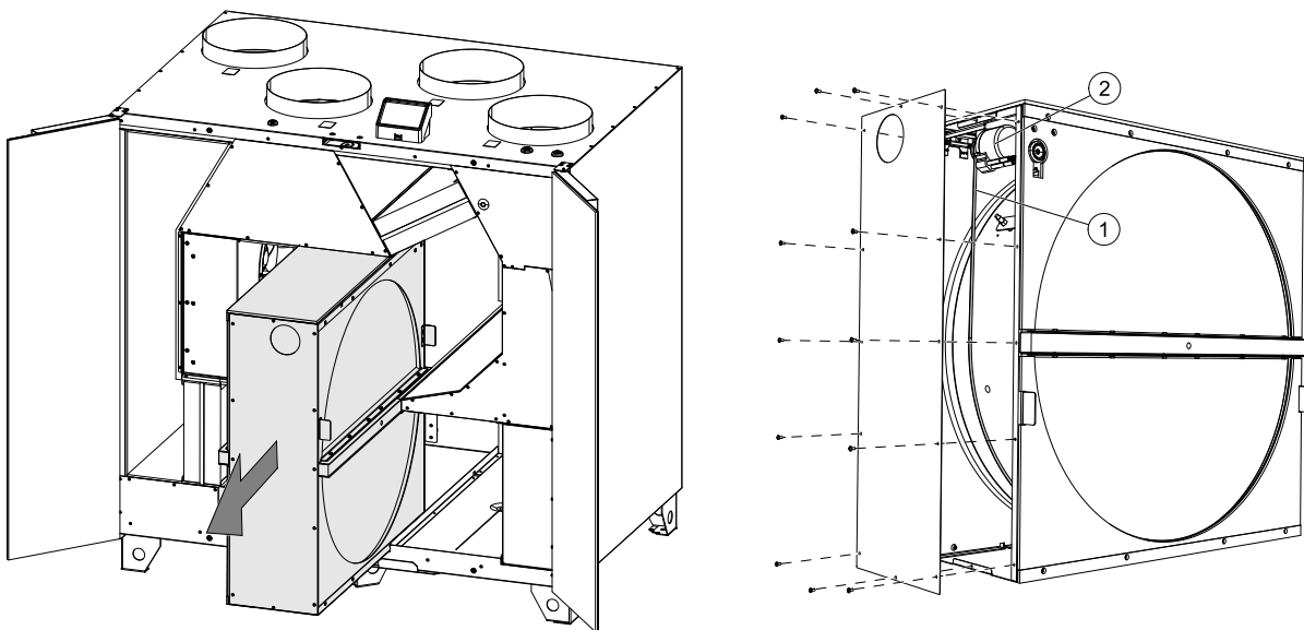
Fig. 7 Toegang tot een gebroken rotor aandrijfriem
