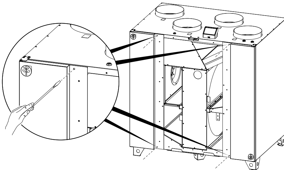
Fig. 4 Zijdeuren openen
