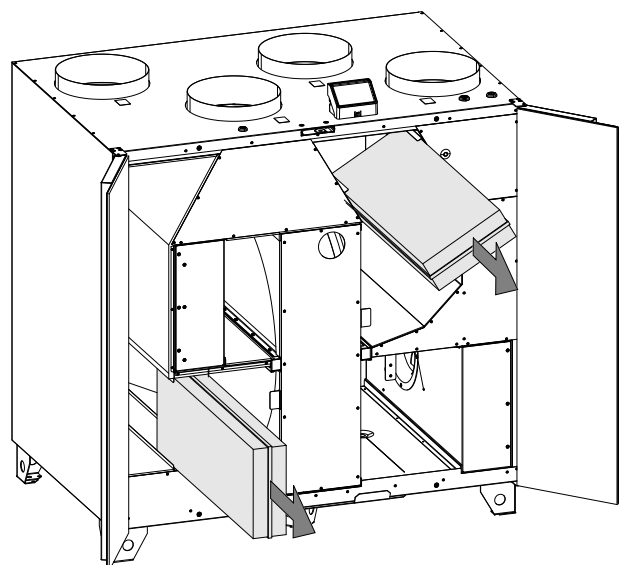
Fig. 5 Filters vervangen
